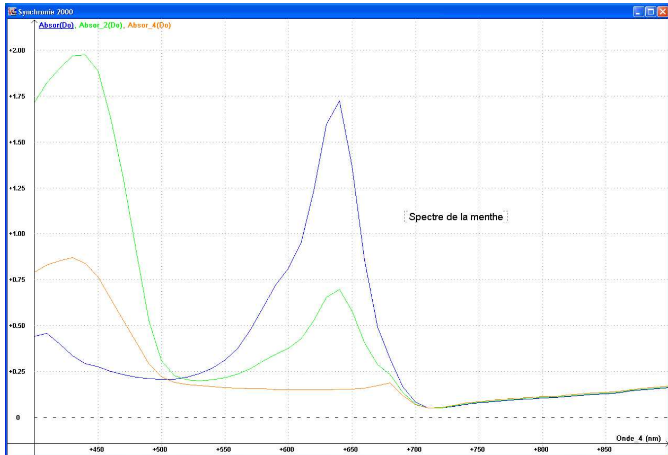
Spectre de la menthe
